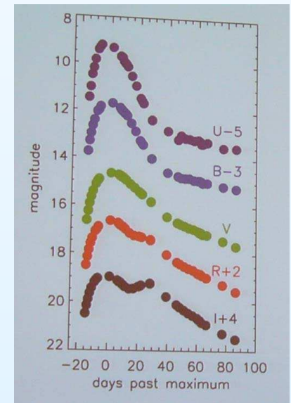
světelné křivky: rozpad ^{56}\text{Ni}
