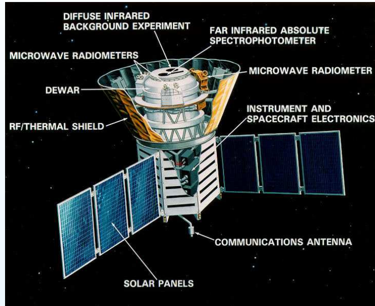
COBE
