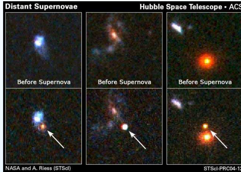
ukázky supernov pozorovaných z HST
