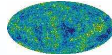
DMR 53 GHz Maps
